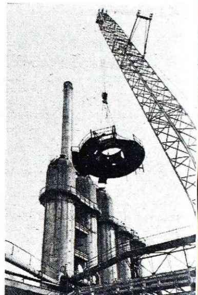
Med remontom plavža 2 (foto S. Kokač)
