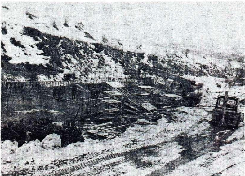
Regulacija potoka Bela (foto S. Kokalj)
