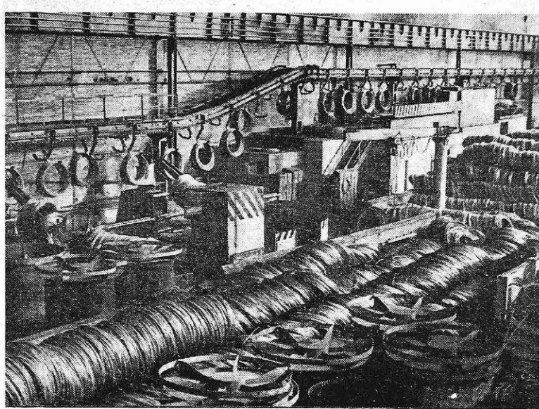
V TOZD Valjarna žice in profilov (foto I. Kučina)
