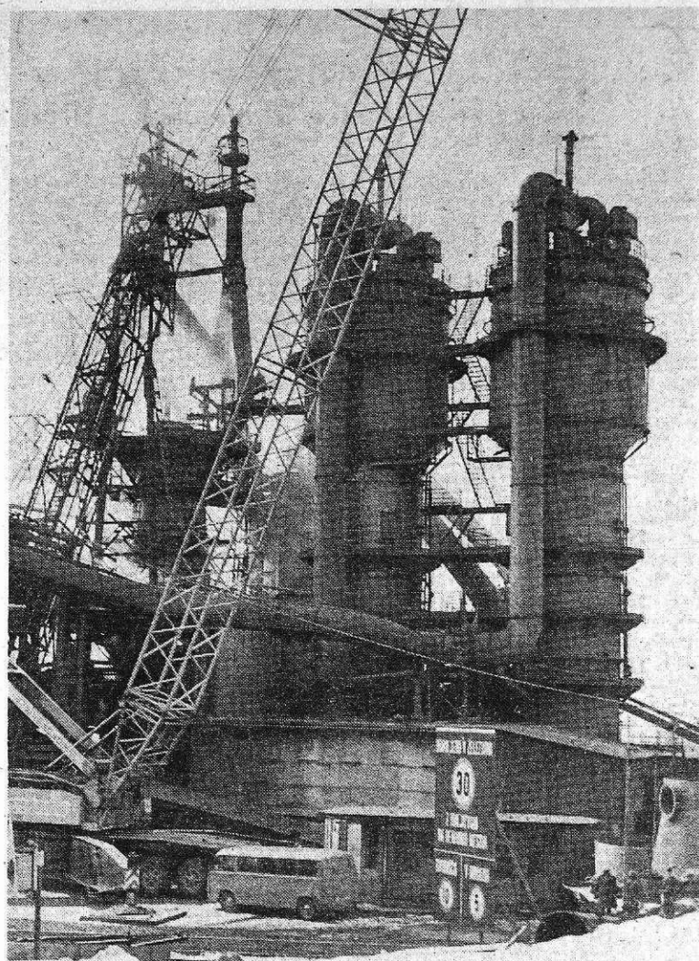
Remont plavža 2 se je pričel 5. marca (foto I. Kučina)
