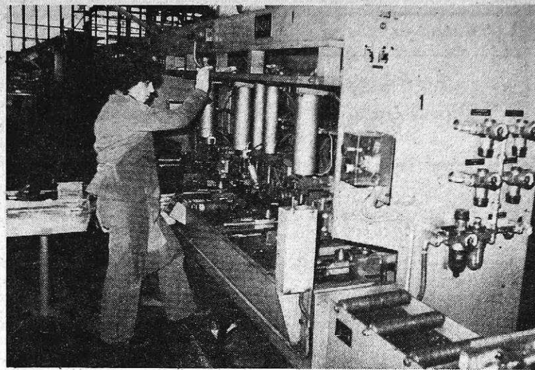
Ob tekočem traku v TOZD Vratni podboji (foto S. Kokalj)
