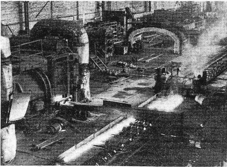
Custudis peč v valjarni žice in profilov (foto I. Kučina)
