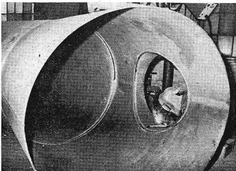
Izdelava cevi za remont Plavža 2 v konstrukcijski delavnici TOZD Strojne delavnice (foto S. Kokalj)
