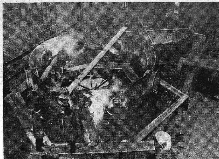
Izdelava plašča za remont Plavža 2 v konstrukcijski delavnici TOZD Strojne delavnice (foto S. Kokalj)
