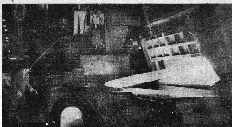
Potisna peč v valjarni debele pločevine (foto I. Kučina)
