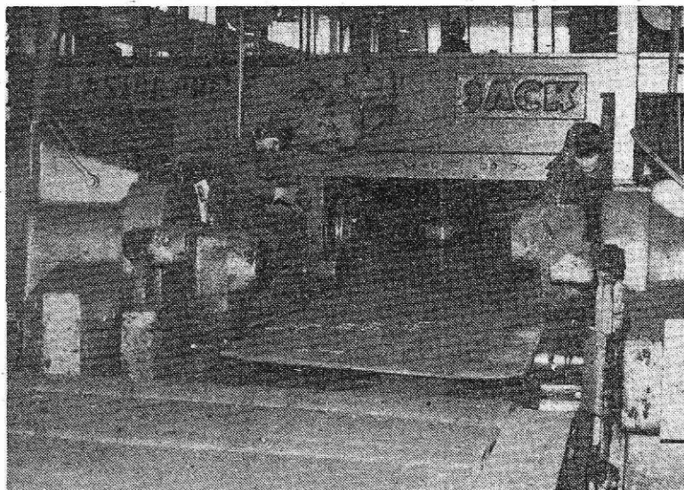
Sodelavca na SACK škarjah v valjarni debele pločevine (foto I. Kučina)
