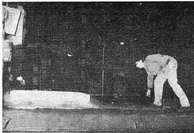
Merjenje debeline v Valjarni debele pločevine (foto S. Kokalj)
