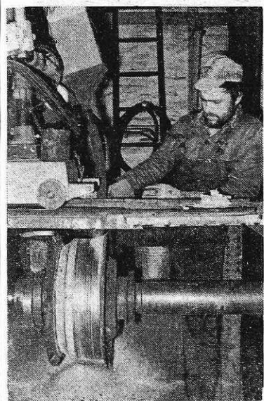
Varjenje pod varilnim praškom v strugarni valjev na Javorniku (foto S. Kokalj)
