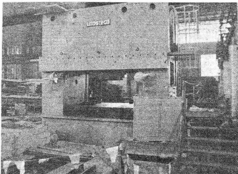
Nova 4000 tonska stiskalnica v TOZD Valjarna debele pločevine (foto I. Kučina)
