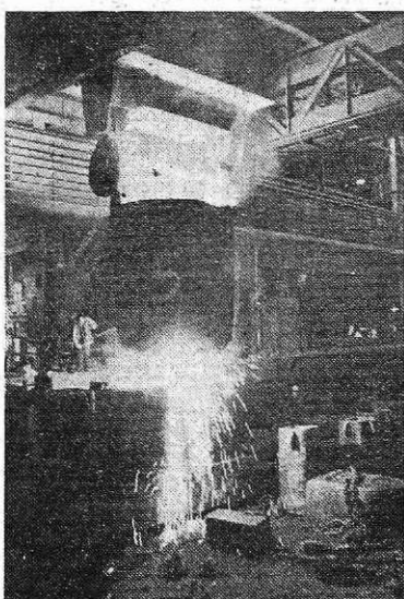
Livna jama v jeklarni (foto I. Kučina)
