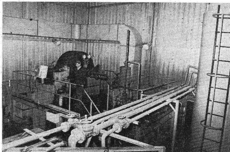
Notranjost objekta regeneracije kislin na Beli (foto S. Kokalj)
