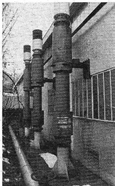
Naprave za zmanjševanje hrupa v kisikarni Sava (foto S. Kokalj)
