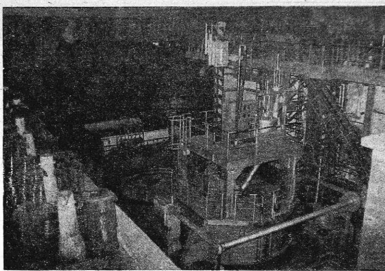
Vakuumska naprava tik pred prvim vročim testiranjem (foto S. Kokalj)
