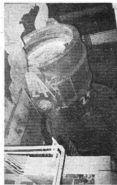
Priprava ponve za vakuumiranje (foto S. Kokalj)
