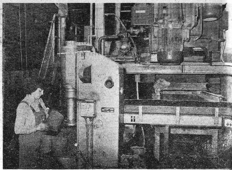
Stiskanje mase za oplašanje elektrod (foto S. Kokalj)
