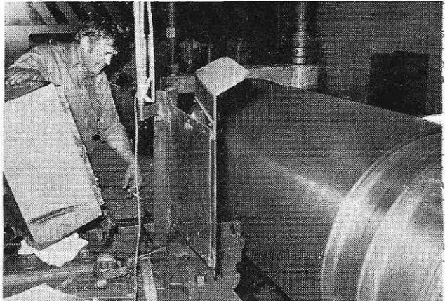
Struženje valja v strugarni valjev na Beli (foto S. Kokalj)
