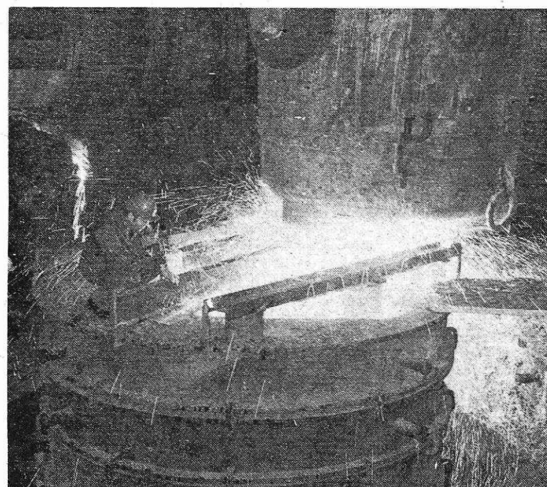
Vlivanje tekočega jekla v kalup iz prve ponve
