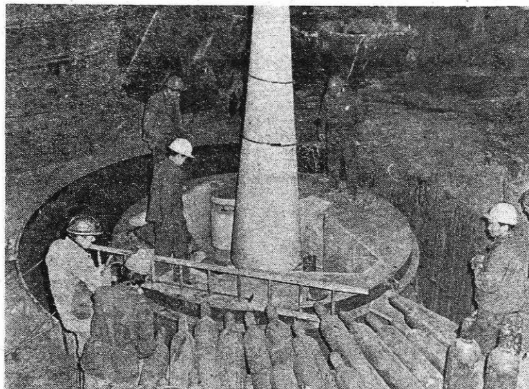
Sestavljanje kalupa za ulitek cilindra
