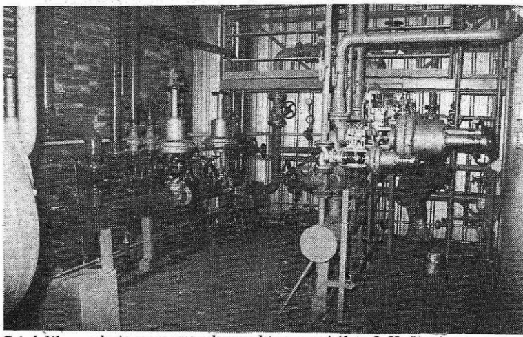
Razdelilec vode in pare na vakuumski napravi (foto I. Kučina)
