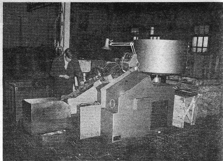
Nov stroj za izdelavo navojnih žebeljev v TOZD Žebeljarna (foto S. Kokalj)
