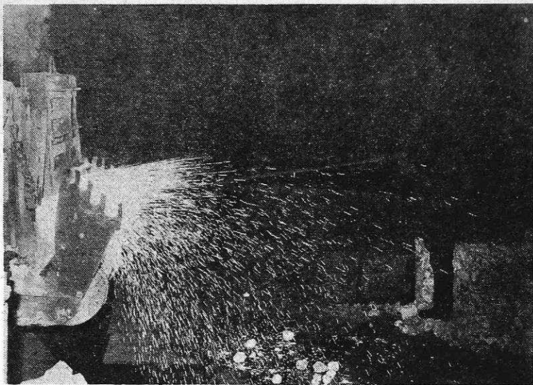
Vpihavanje v BBC električno peč (foto S. Kokalj)
