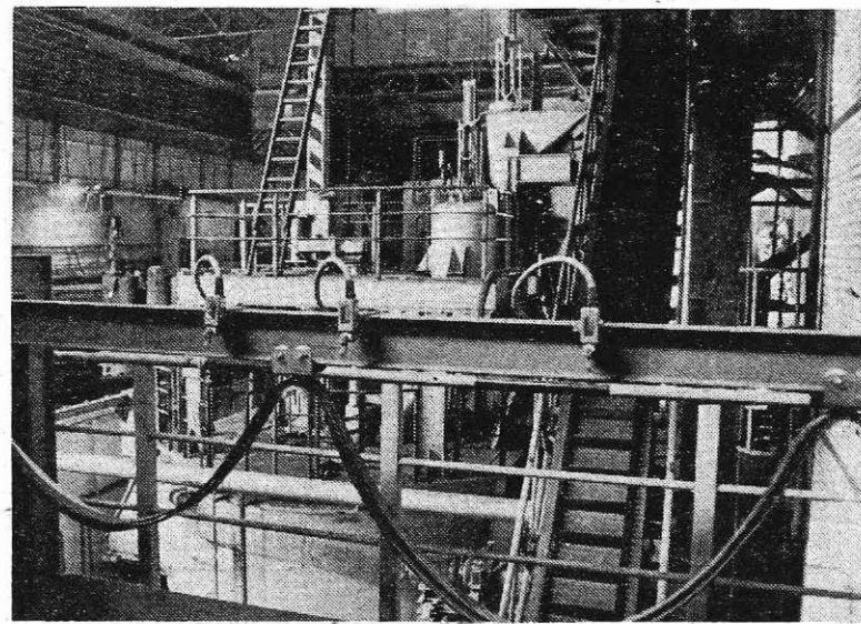
Vakumska naprava v jeklarni (foto I. Kučina)
