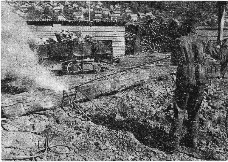
Rezanje »svin« na nasipu (foto I. Kučina)
