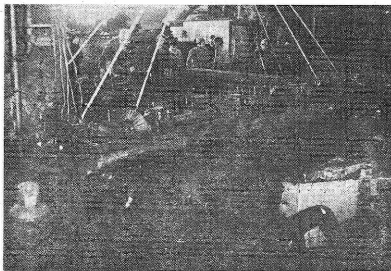
Montaža valjčnega ogrodja v valjarni debele pločevine (foto S. Kokalj)
