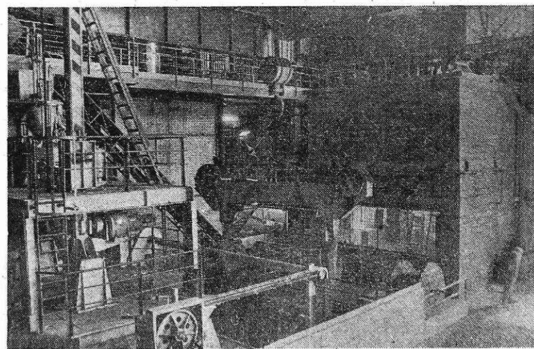
Sestav naprav za vakumiranje jekla (foto I. Kučina)
