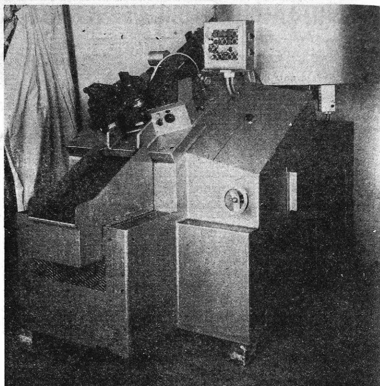
Stroj za valjanje žebeljev — Iw-3-8
