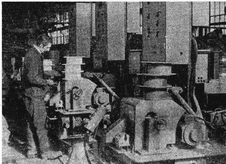
Izdelava VAC žice v TOZD Žičarna (foto I. Kučina)
