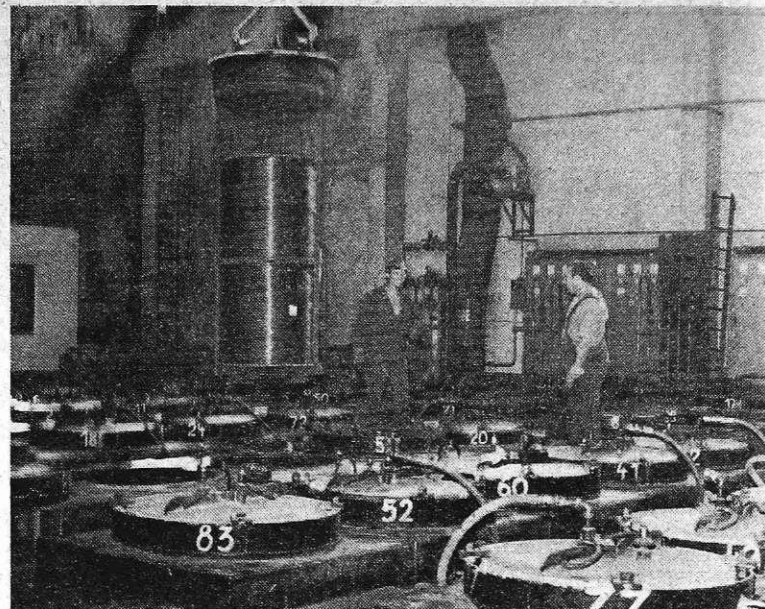
Zvonaste peči v Žičarni (foto I. Kučina)
