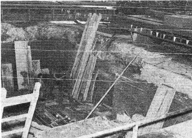
Temelji za nov 4.000-tonski ravnalnik v valjarni debele pločevine (foto I. Kučina)
