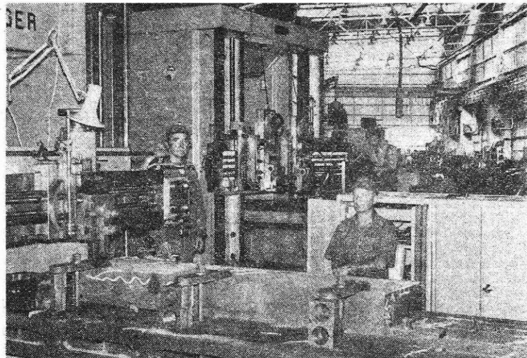
Strojne delavnice, težka obdelava na Javorniku (foto I. Kučina)
