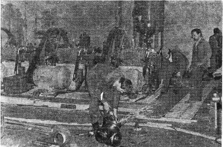
Montaža naprav za odbrizg kovarine v strojnici valjarne debele pločevine (foto I. Kučina)
