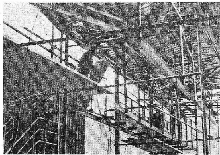
Del vakumske naprave — montaža (foto I. Kučina)
