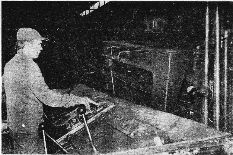
Linija za rezanje pločevine v valjarni bluming štekel (foto I. Kučina)
