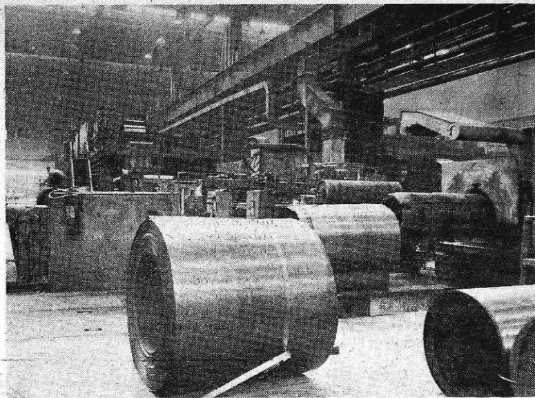
Izstopni del žarilne linije v hladni valjarni Bela (foto I. Kučina)
