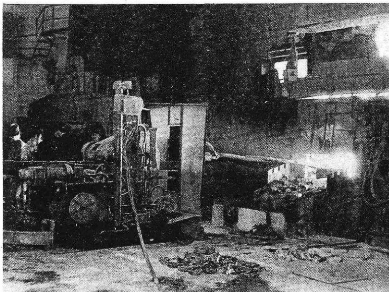
ASEA električna peč med obratovanjem (foto I. Kučina)
