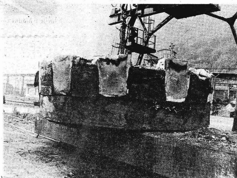
Vlitek nosilnega prstana za tovarno Djuro Djaković (foto S. Kokalj)
