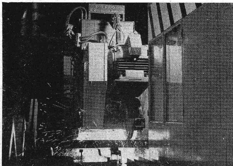
BSG 4000 — nov brusilni stroj, izdelan v železarni (foto I. Kučina)
