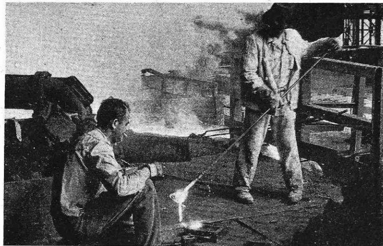
Odzem poskusnega vzorca na Plavžu (foto I. Kučina)
