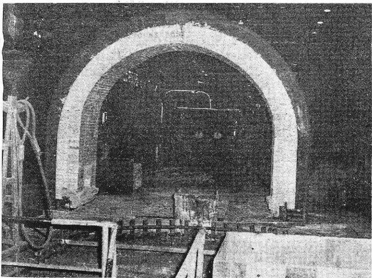
Rezervni obok Custodis peči v valjarni žice (foto S. Kokalj)
