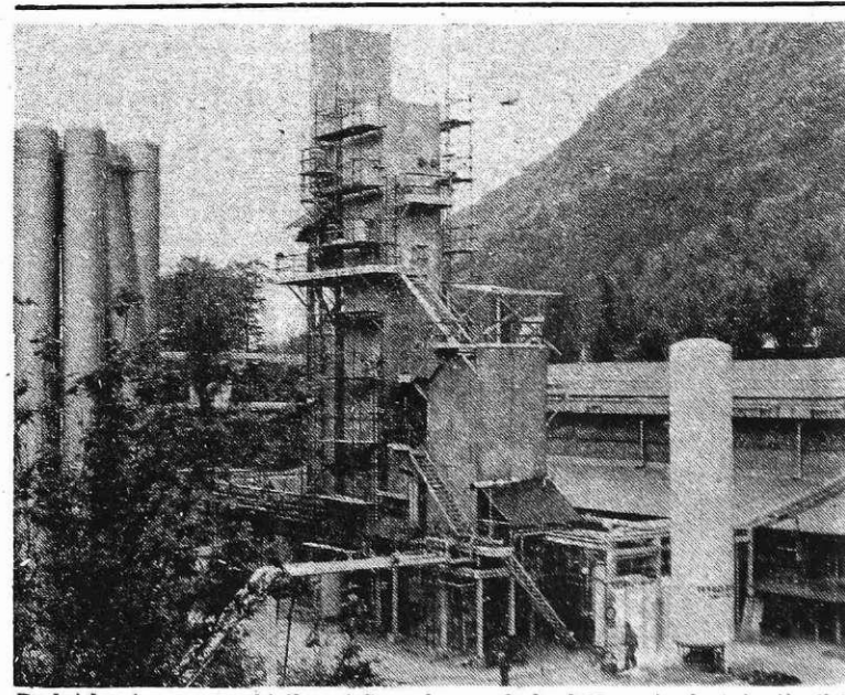
Redni letni remont v kisikarni Sava bo potekal od 15. maja do 1. junija (foto I. Kučina)
