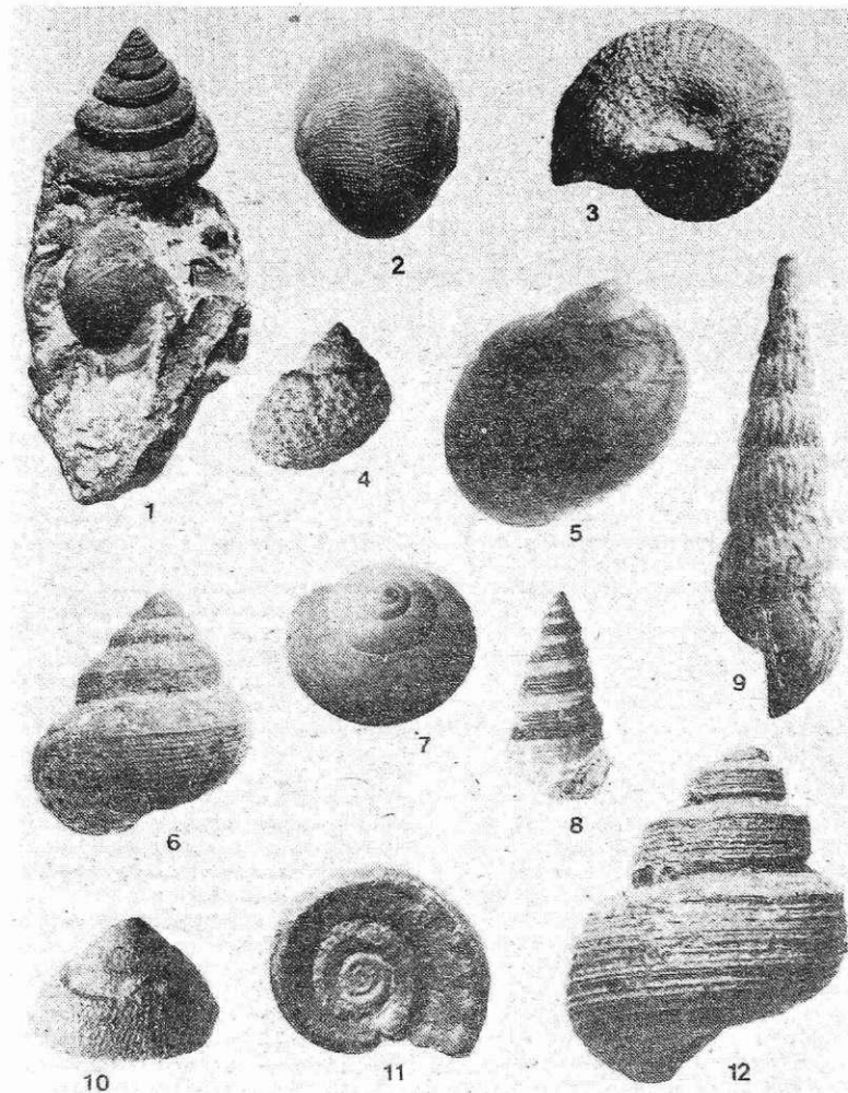
Okameneli morski polži iz spodnjepermijskih kamnin na Pristavi (starost okrog 280 milijonov let): 1. LOPHOSPIRA sp., 2. BELLEROPHON GRAFHICUS, 3. BELLEROPHON sp., 4. TRACHYDOMIA NODOSA, 5. NATICOPSIS ORNATA, 6. WORTHENIA sp., 7. ANOMPHALUS sp., 8. STEGOCOELIA sp., 9. PSEUDOZYGOPELEURA sp., 10. AMOURLONIA sp., 11. STRAPAROLUS PERNODOSUS, 12. BAYLEA sp. (foto J. Bedič)
