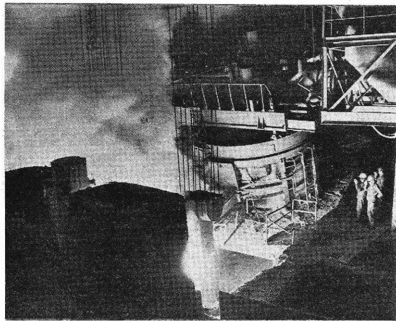
Prebod na Lectromelt električni peči (Foto I. Kučina)
