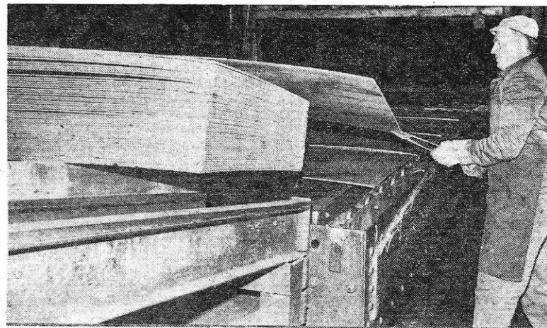
Custodis normalizirna peč v valjarni na Javorniku (foto I. Kučina)
