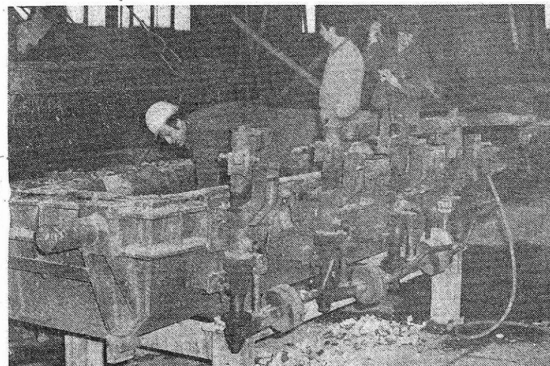
Čiščenje vmesne ponve za vlivanje na kontilivu (foto S. Kokalj)
