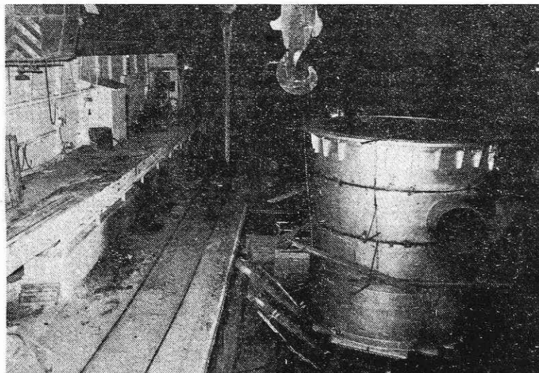
Vakuumska komora na vakuumski napravi (foto I. Kučina)
