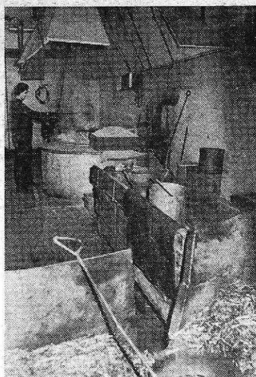
Pocinkovalnica žičnikov (Foto I. Kučina)
