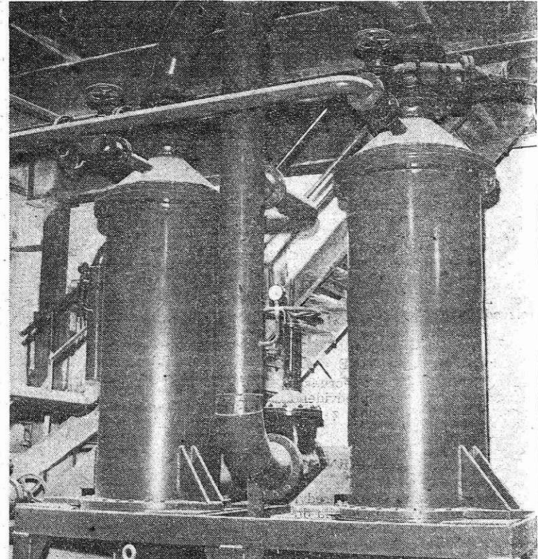
Nova filtrska postaja hladilne vode za Lectromelt električno peč
