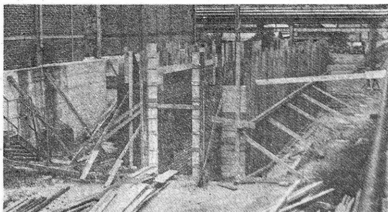
Začetek gradnje podaljška hale valjarne težke pločevine lansko jesen
