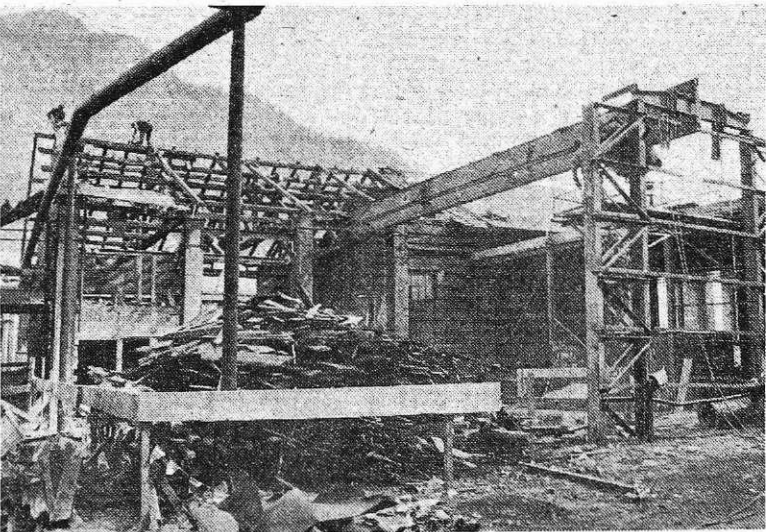
Adaptacija stare lužilnice za razširitev delavnice za motorna vozila (Foto I. Kučina)
