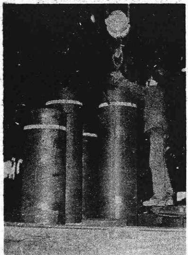
Menjava elektrod na Lectromelt električni peči (foto I. Kučina)
