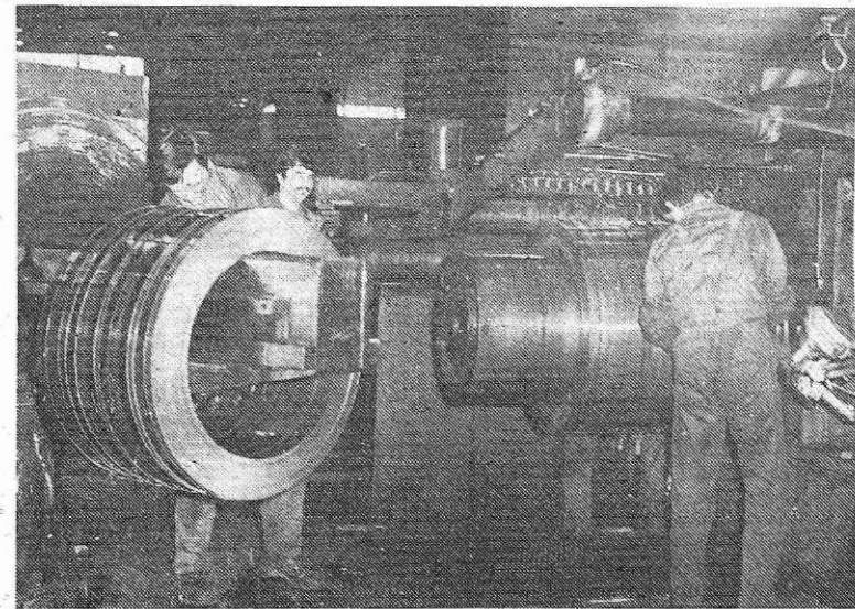
Izdelava trakov za povezovanje pločevine (Foto S. Kokalj)
