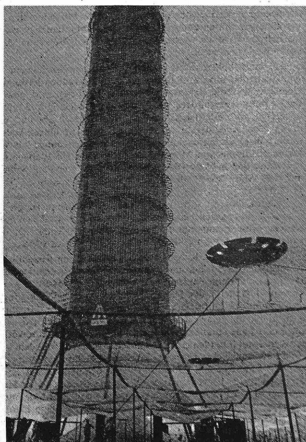
Pogled na streho iz folije in del kamina naprave v Manzaresu.
