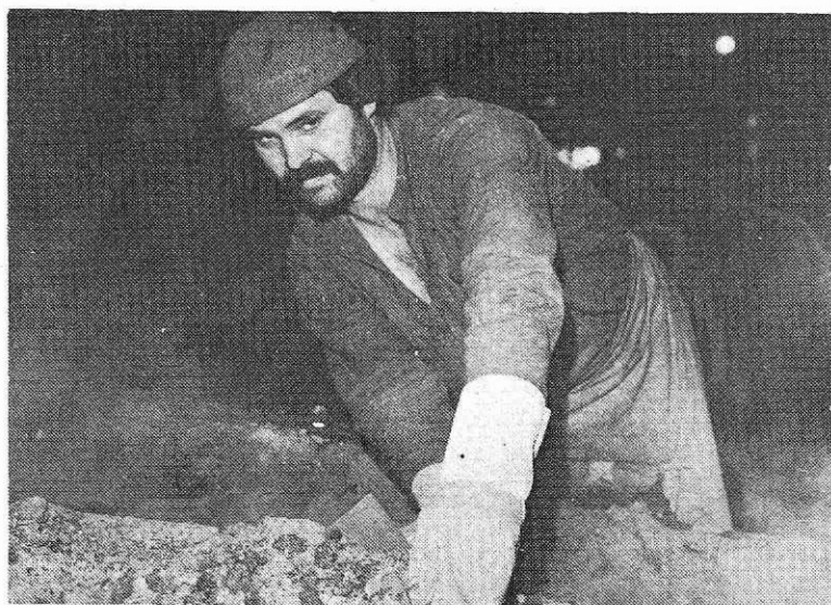
Obzidava livnega žleba pri SM peči (Foto I. Kučina)
