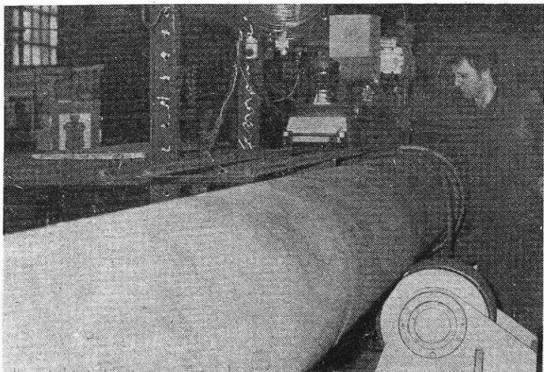
Avtomatsko navijanje vretena v konstrukcijski delavnici (Foto S. Kokalj)
