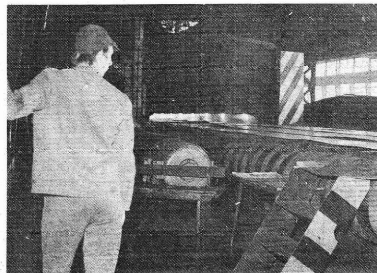
Custodis normalizirna peč v valjarni debele pločevine (Foto I. Kučina)
