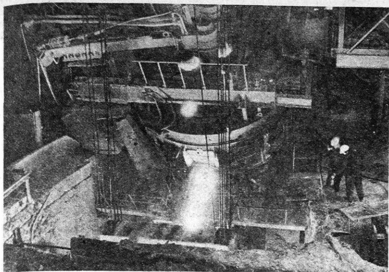
Sarž na Lectromelt električni peči (Foto I. Kučina)
