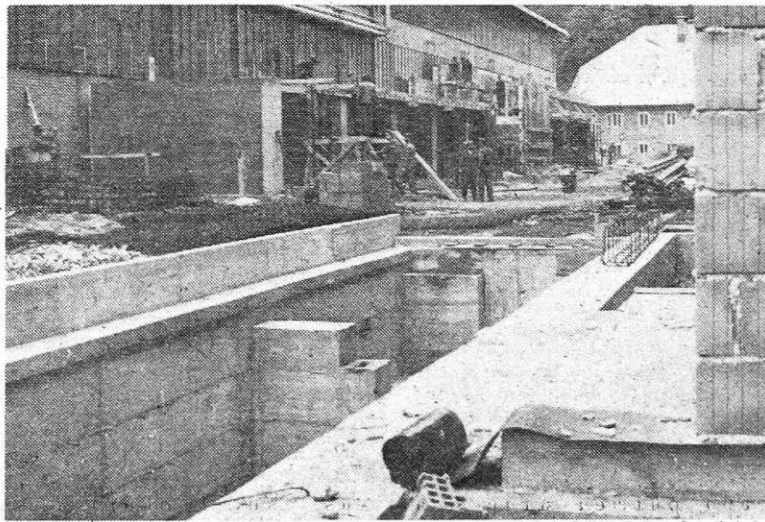
Temelji za novo železniško tehniko na Javorniku (Foto I. Kučina)
