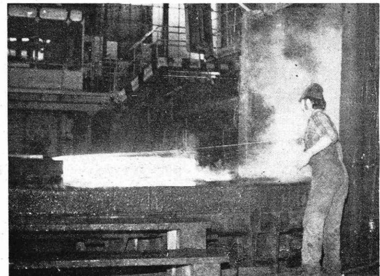
Valjanje debele pločevine (Foto I. Kučina)
