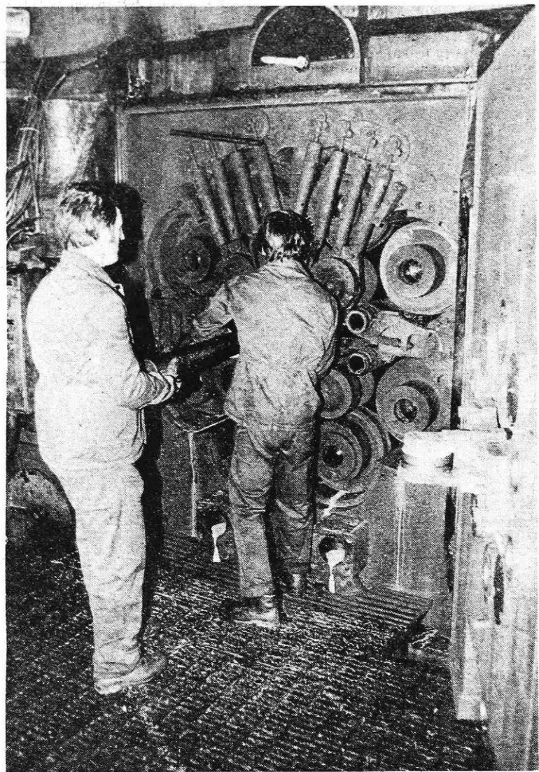
Menjava valjev na Sendzimir ogrođu (Foto S. Kokalj)
