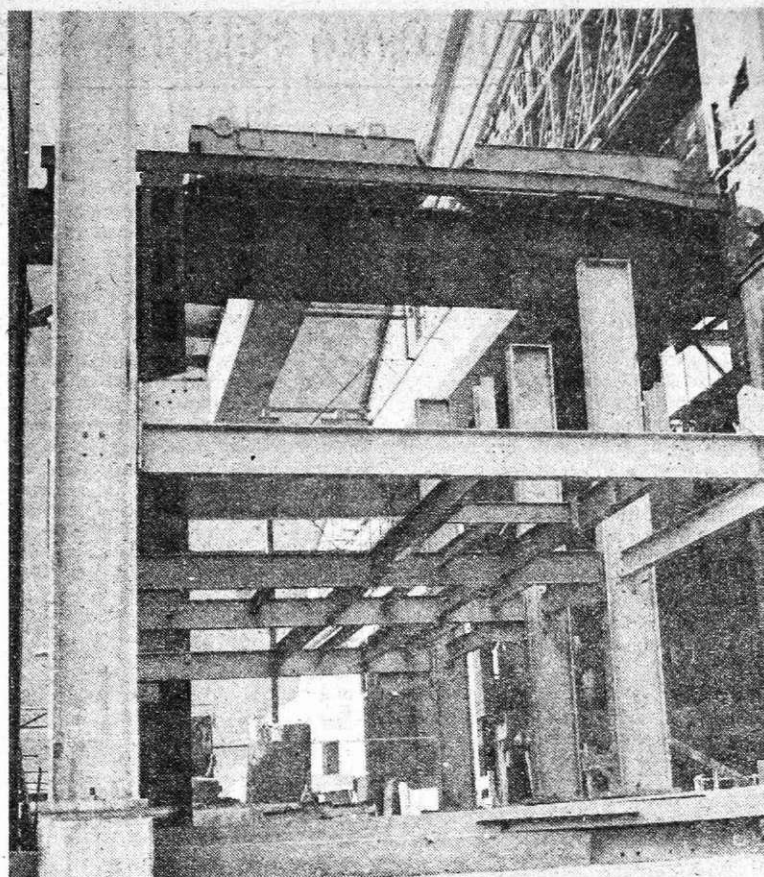
Gradnja vakumske naprave (Foto I. Kučina)
