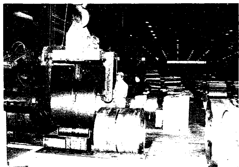
V hladni valjarni Bela (Foto S. Kokalj)
