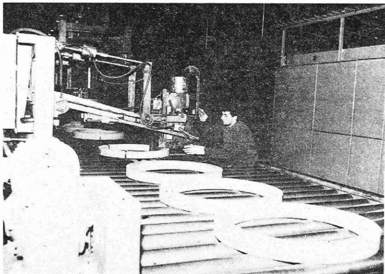
Automatsko povezovanje travok (Foto S. Kokalj)
