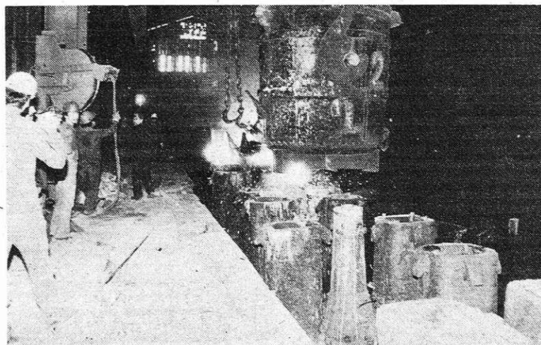
Vlivanje jekla (Foto S. Kokalj)
