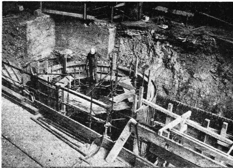
Gradnja vakumske komore (Foto I. Kučina)
