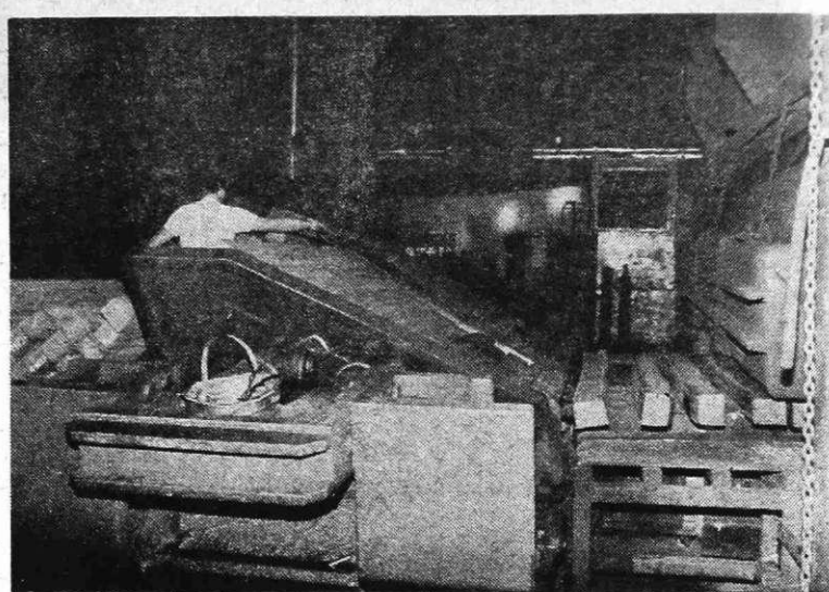
Zakladanje peči v valjarni žice na Beli (Foto I. Kučina)
