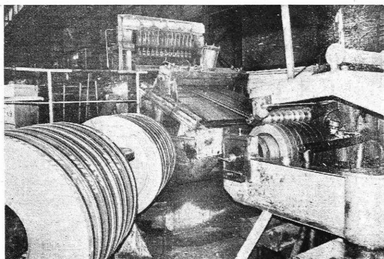
Bronx škarje v valjarni Bela (Foto I. Kučina)
