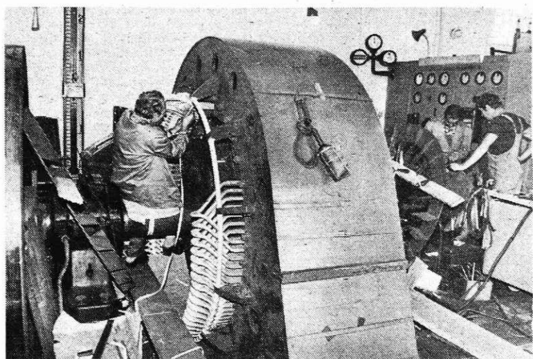
Obnova generatorja hidrocentrale v Zapisu poteka natančno po planu. Delavci Elektromonta iz Subotice hitijo, da bomo lahko izkoristili jesenske vode. (Foto I. Kučina)
