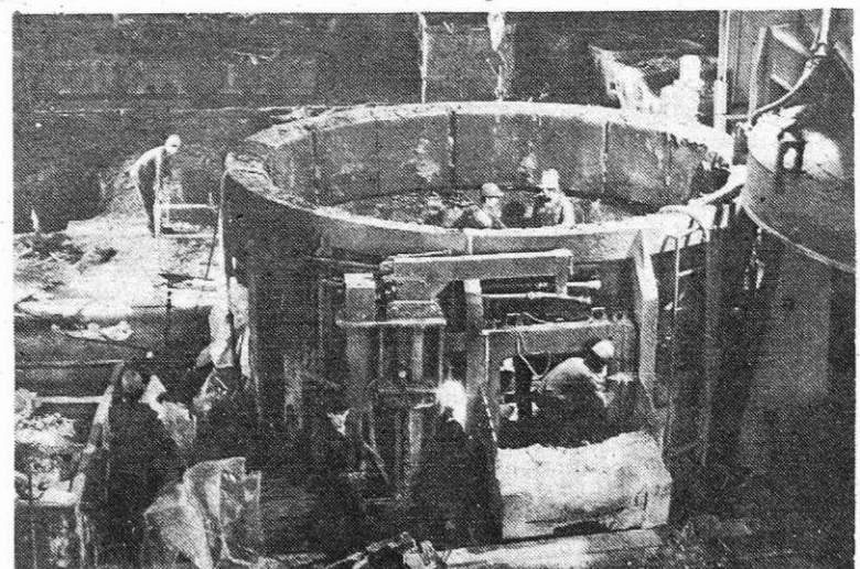
Enodnevni remont na Lectromelt električni peči (Foto I. Kučina)
