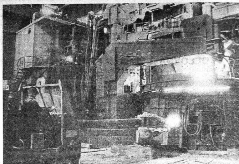
Dodajanje materialov v ASEA električno peč (Foto I. Kučina)
