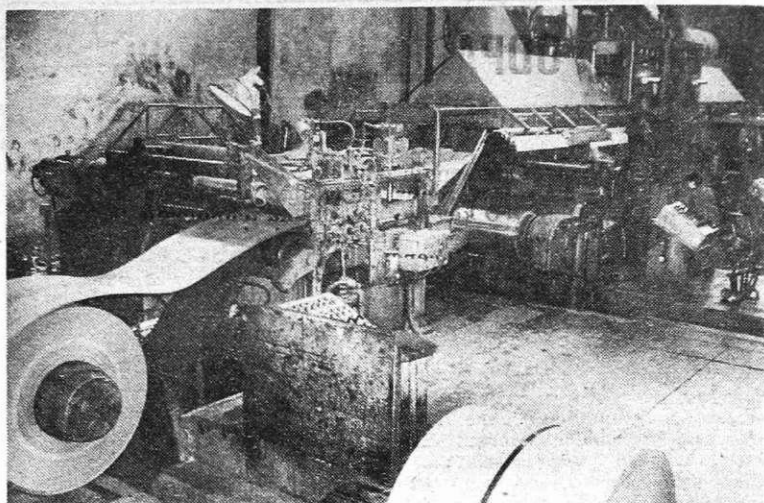
Sendzimir ogrodje v hladni valjarni Bela (Foto I. Kučina)
