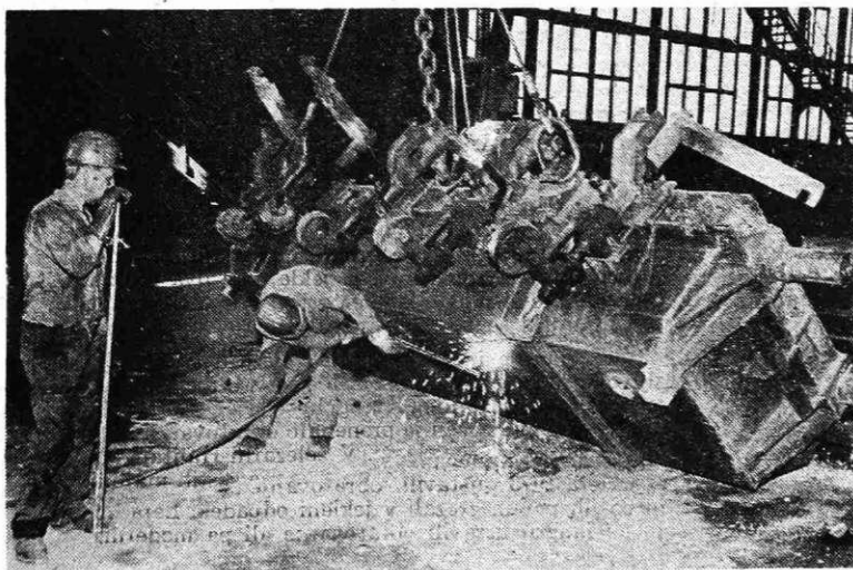
Čiščenje umesne ponve v konti livu (Foto I. Kučina)
