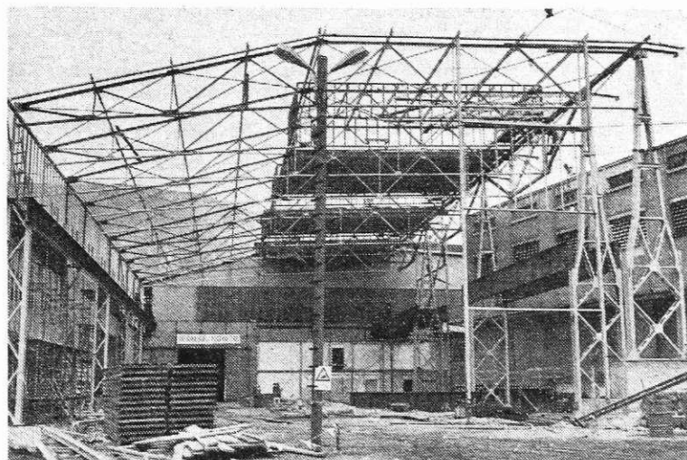
Konstrukcija podaljška hale valjarne debele pločevine (Foto I. Kučina)
