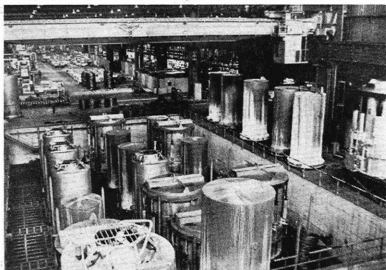
Zvonaste peči v hladni valjarni Bela (Foto I. Kučina)
