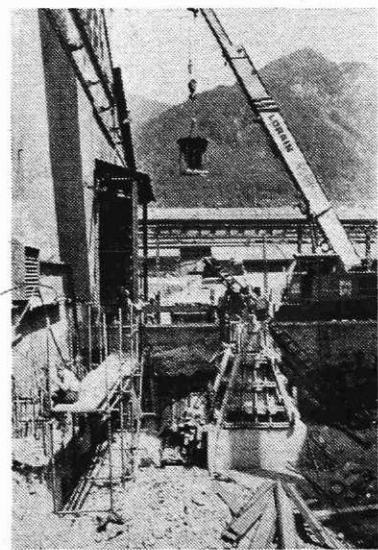
Betoniranje podaljška hale za novo vakuumsko napravo (Foto I. Kučina)
