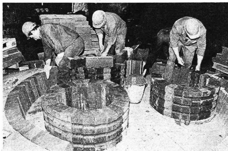
Industrijski zidarji obzidavajo pokrove za električno peč (Foto I. Kučina)
