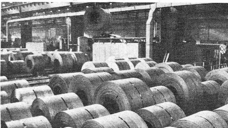
V hladni valjarni Bela (Foto I. Kučina)
