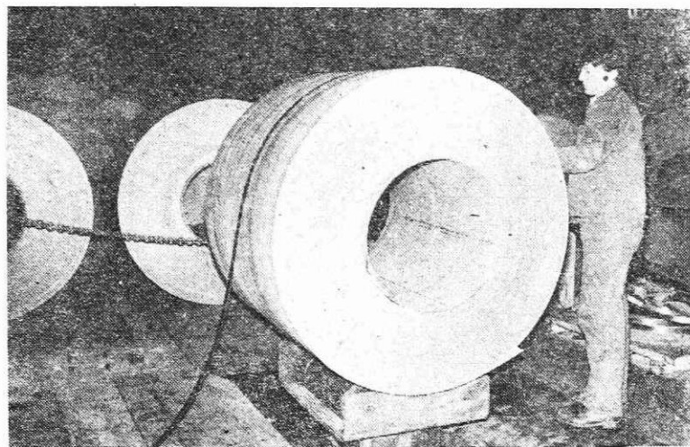
Izstopni del žarilno-lužilne linije v hladni valjarni Bela (Foto I. Kučina)
