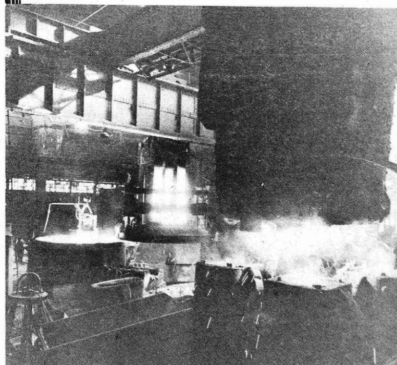
Vlivanje jekla (Foto I. Kučina)
