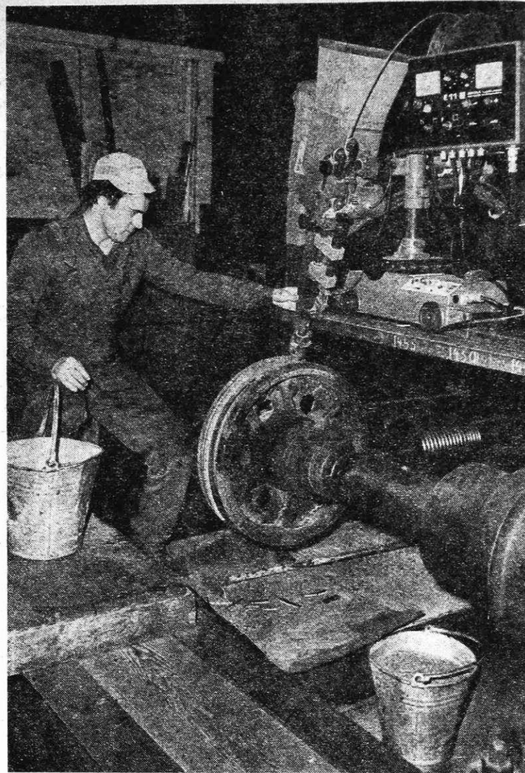
Automatsko varjenje pod varilnim praškom v strugarni valjev (Foto S. Kokalj)
