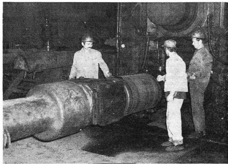
Menjava delovnih valjev na ogrodju štekel (Foto S. Kokalj)
