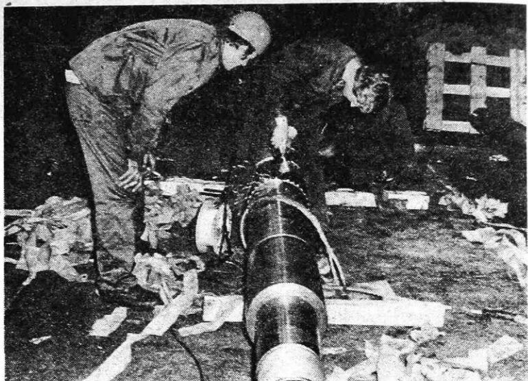
Priprava gredi odvajalca pred montažo ob remontu na Sendzimir ogrođju (Foto S. Kokalj)
