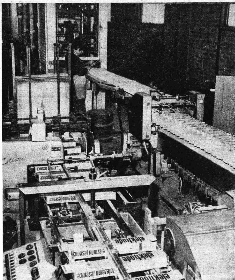
Kontrola in strojno pakiranje elektrod (Foto I. Kučina)
