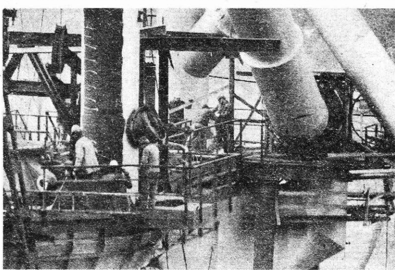
Remont plavža številka 1 (Foto I. Kučina)
