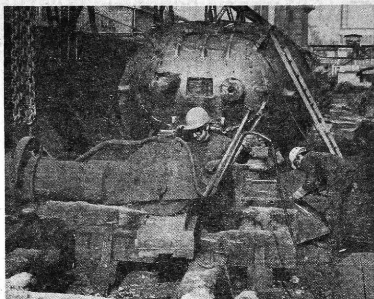
Sodelavca pri čiščenju odlitkov v sivi livarni (Foto I. Kučina)
