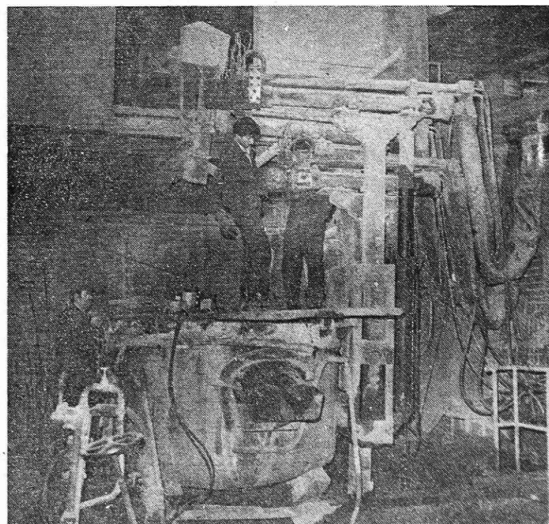
Remont točilne peči za elektrodni prašek (Foto I. Kučina)
