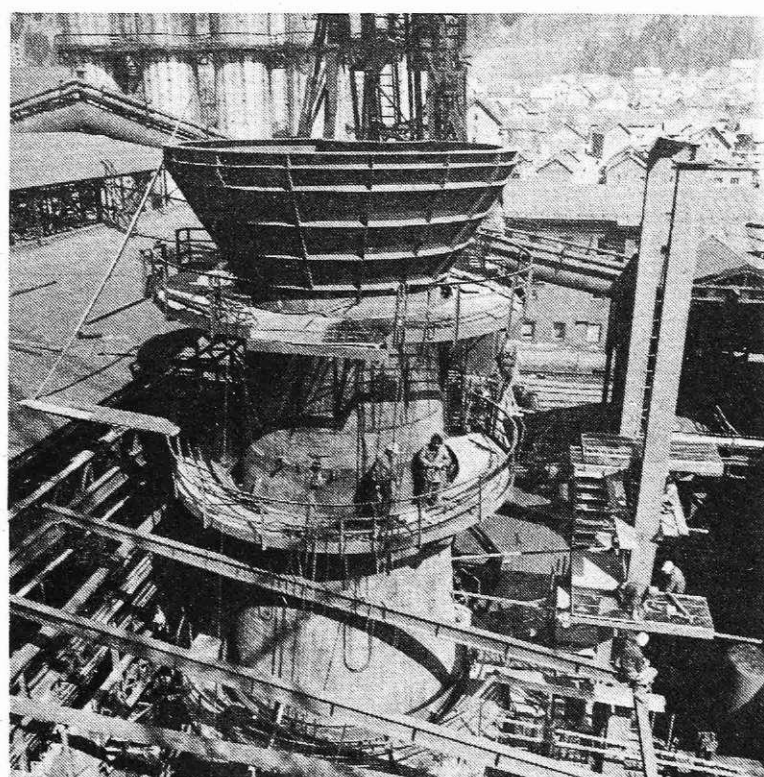
Remont na plavžu 1 (Foto I. Kučina)
