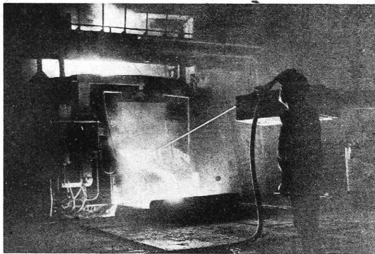
Vpihavanje kisika v električno peč (Foto I. Kučina)
