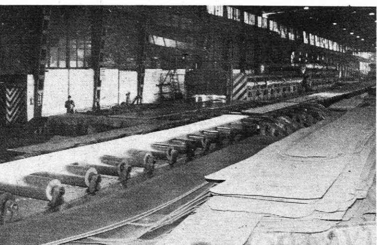
V valjarni debele pločevine (Foto I. Kučina)
