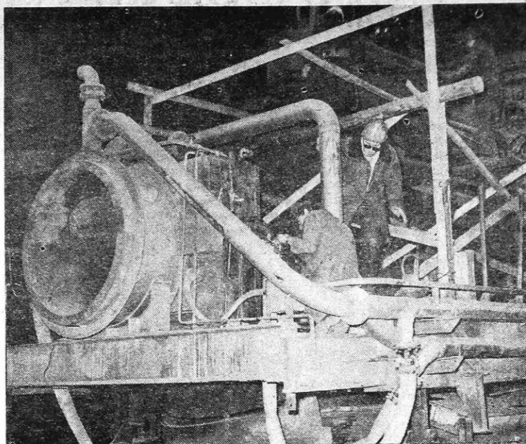
Remont na Lectromelt električni peči (Foto I. Kučina)
