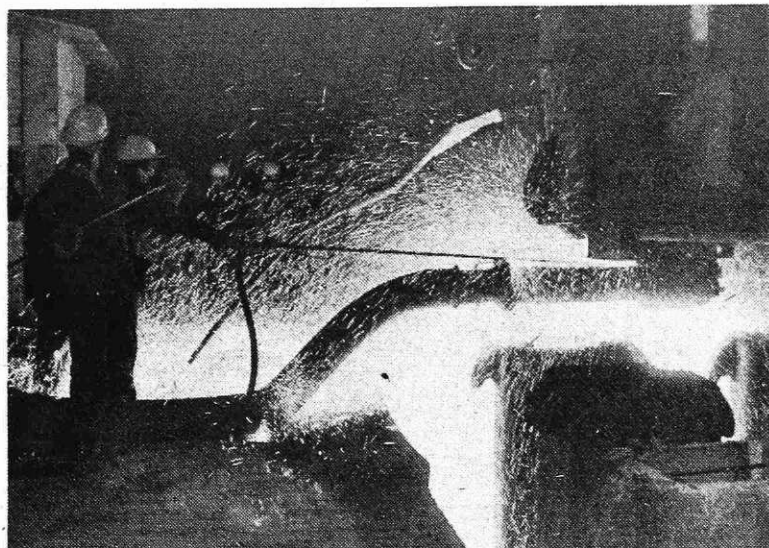
Ulivanje v elektro jeklarni (Foto I. Kučina)
