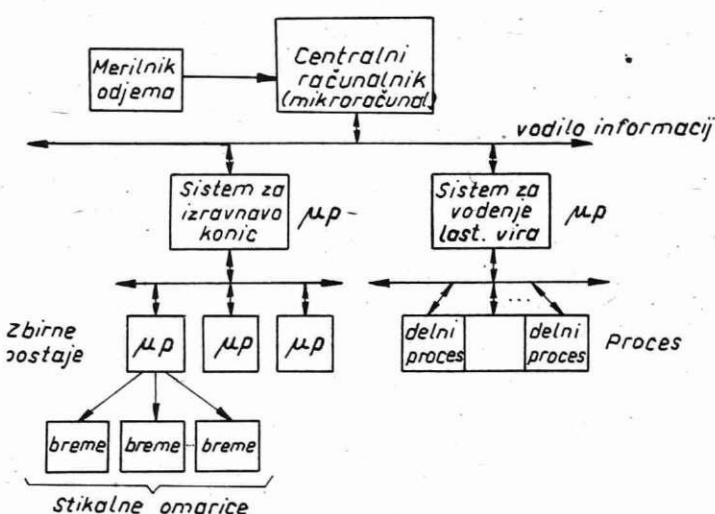
Slika 16: Sistem za vodenje energetske situacije v podjetju z vključitvijo lastnega vira
