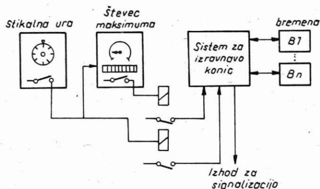
Slika 14: Shema povezave sistema za izravnavo konic
